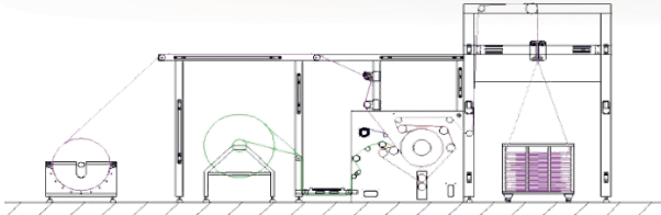
Şekil 1. Film Laminasyon Makinesi
