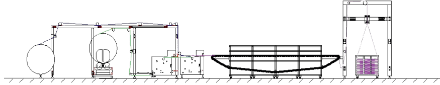
Şekil 2. Laminasyonlu Kaymaz Taban Halı Hattı
